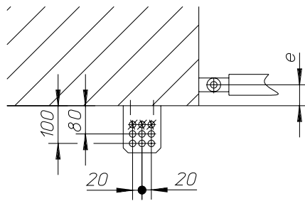
Ausführung "Lang"
