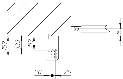
Ausführung "Normal"
