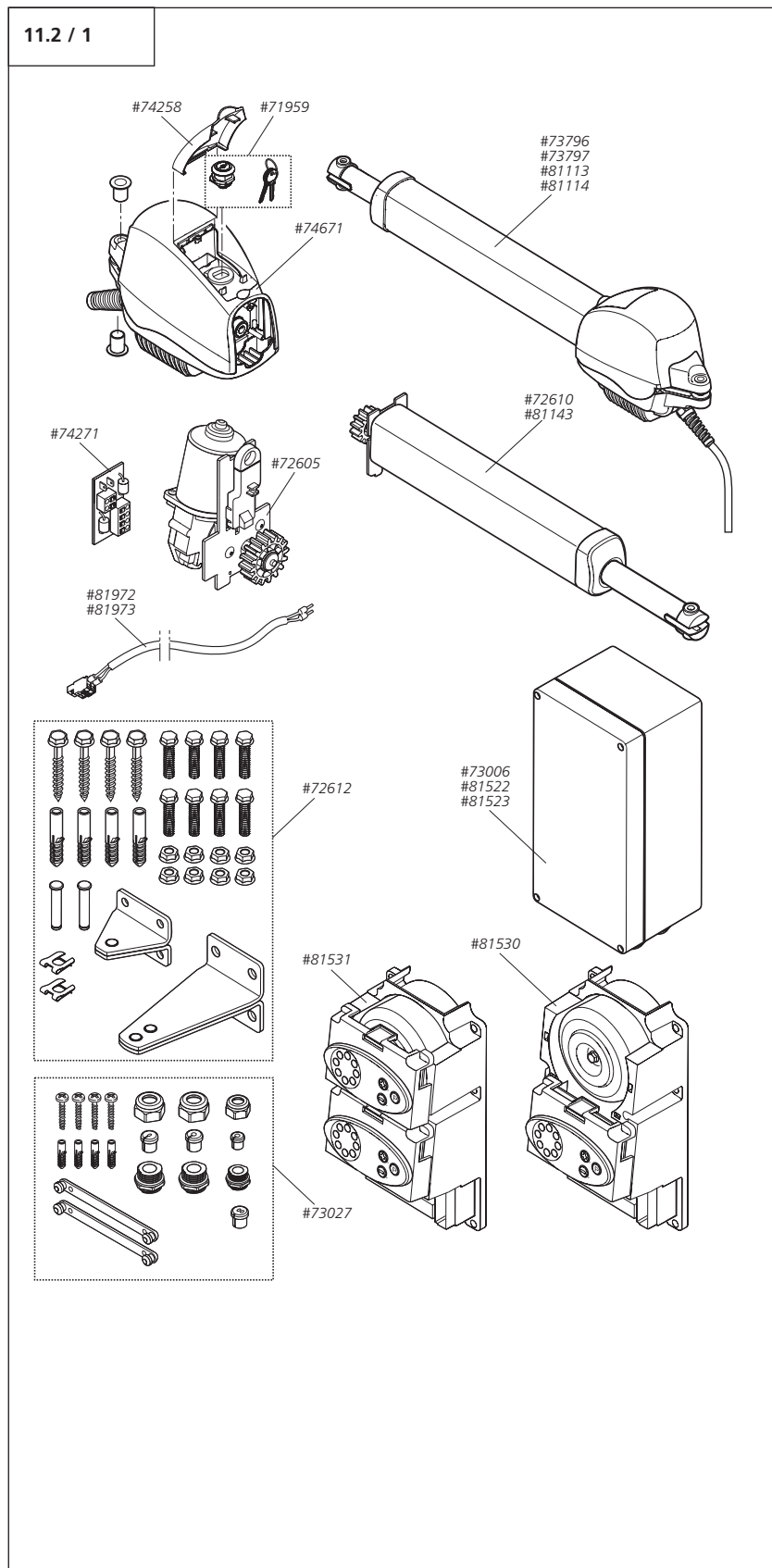
Legende Ersatzteile 11.2 / 1
