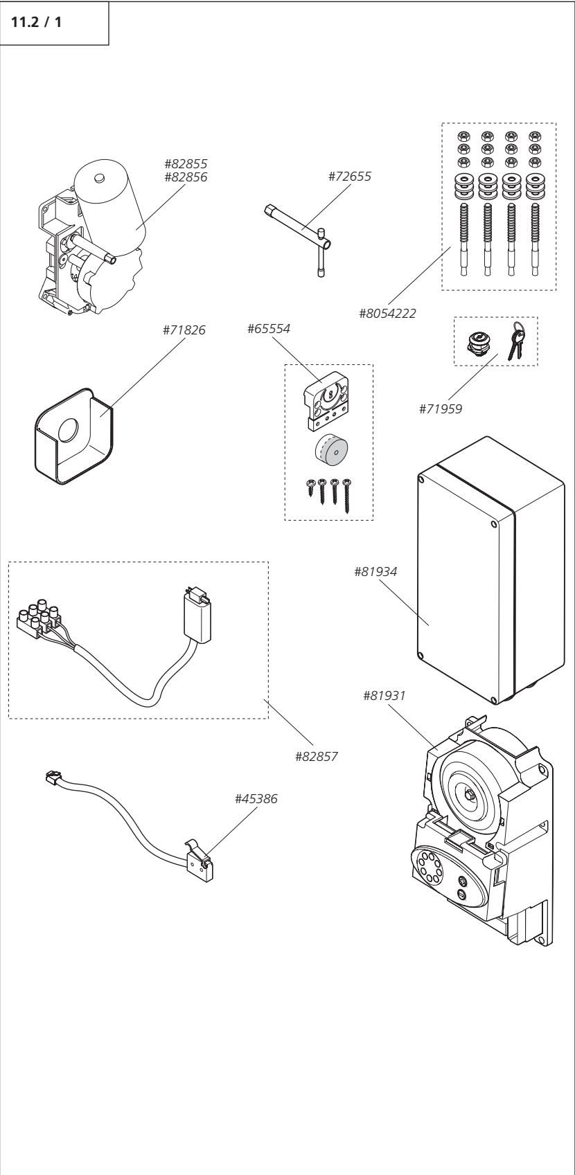
Legende Ersatzteile 11.2 / 1
